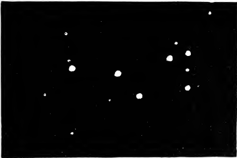
Fig. 87.—The Pleiades.
